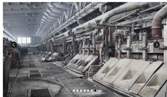
Aluminij pridobivamo z elektro-kemičnim procesom v elektroliznih pečeh, kje se glinica razkaja na svoje komponente, aluminij in kisik. Proces poteka v raztopini elektrolita pri temperaturi od 950 do 970 °C.
